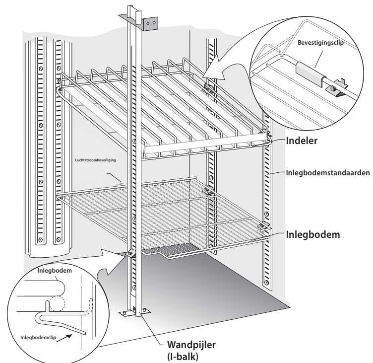
Afb. 5. Close-up van een inlegbodem op inlegbodemclips en de bevestigingsclips.
