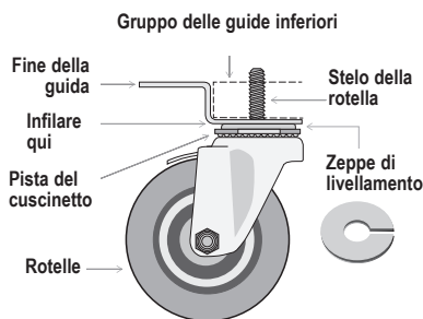
Fig. 7 Diagramma della rotella orientabile.
