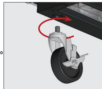
Fig. 8 Avvitare le rotelle orientabili nei fori filettati.
